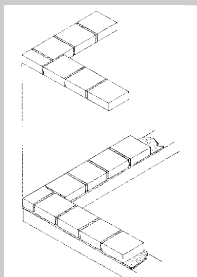
Aparejados de muros en forma de "L", aparejado de la primera y segunda hiladas
