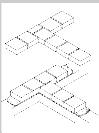
Aparejados de muros en forma de "T", aparejado de la primera y segunda hiladas
