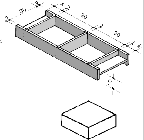
Adobe entero: 30x30x10
