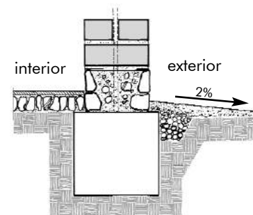
Sobrecimiento encofrado con piedras y relleno de hormigón.
