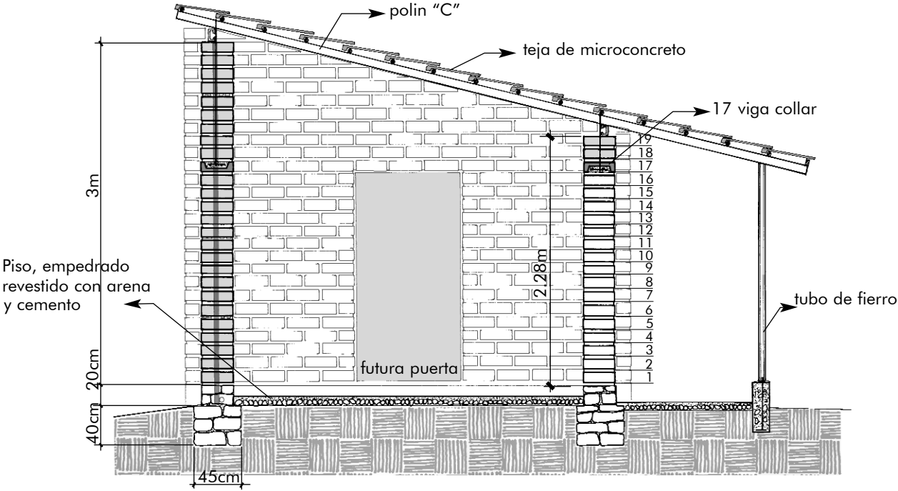
CORTE A-A
