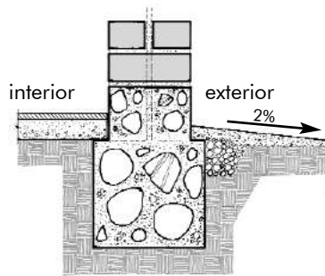
Cimiento de hormigón ciclópeo
