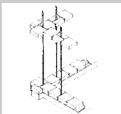
Aparejados de muros en esquina, con refuerzos verticales
