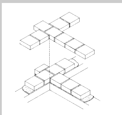
Aparejados de muros en intermedios, con contrafuertes
