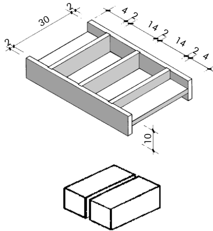
1/2 Adobe: 30x14x10
