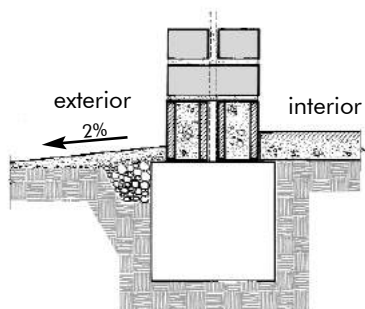
Sobrecimiento con bloques de hormigón (40x20x14cm) y relleno con hormigón.
