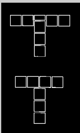
Aparejados de muros en forma de "T", aparejado de la primera y segunda hiladas
