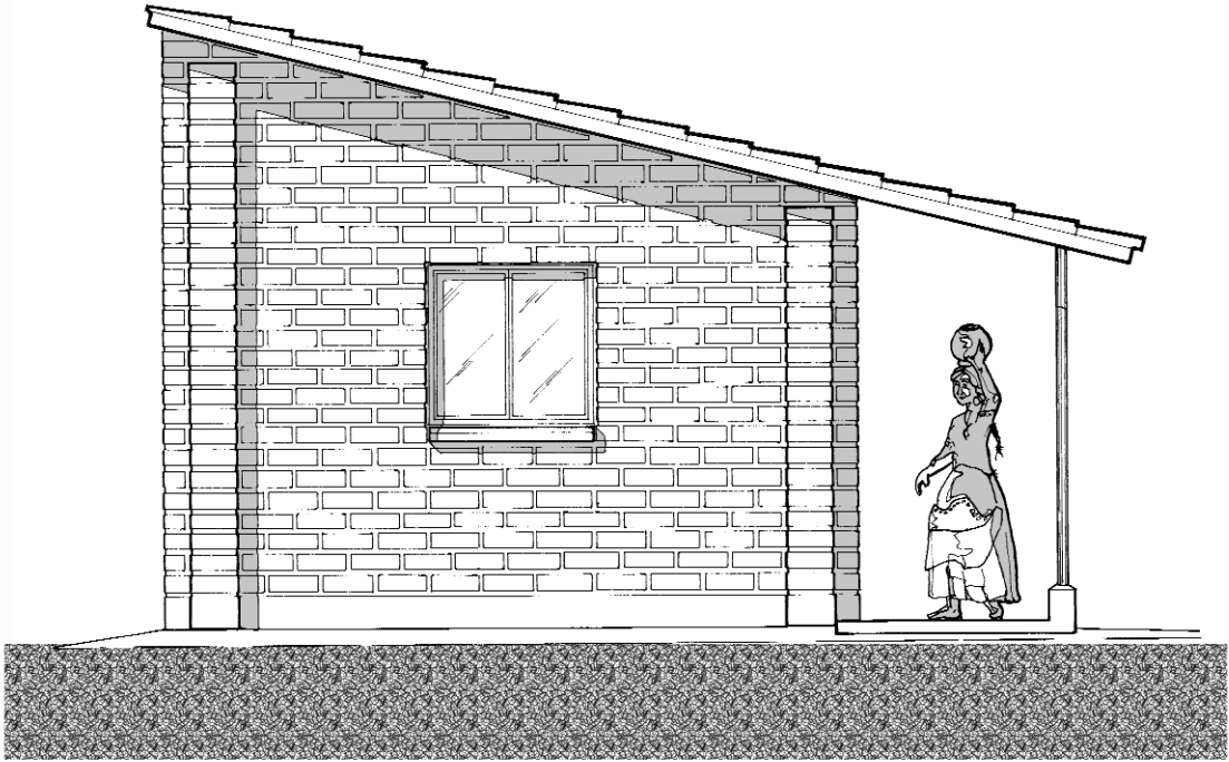
ELEVACION LATERAL IZQUIERDA
