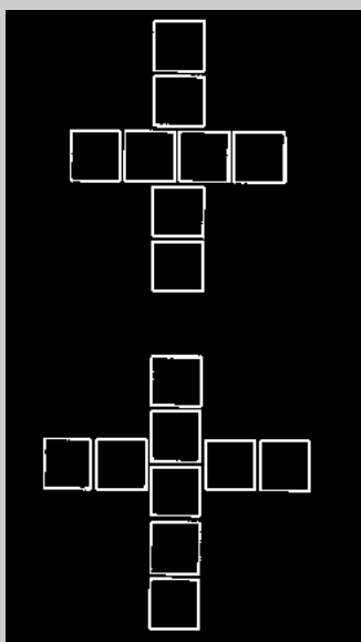
Aparejados de muros en forma de "+", aparejado de la primera y segunda hiladas
