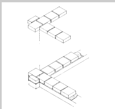
Aparejados de muros en esquina, con contrafuertes
