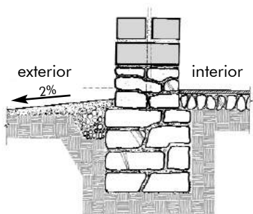
Cimiento de mampostería de piedra
