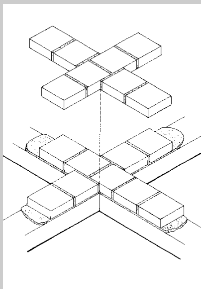
Aparejados de muros en forma de "+", aparejado de la primera y segunda hiladas
