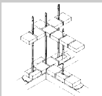
Aparejados de muros en intermedios, con refuerzos verticales
